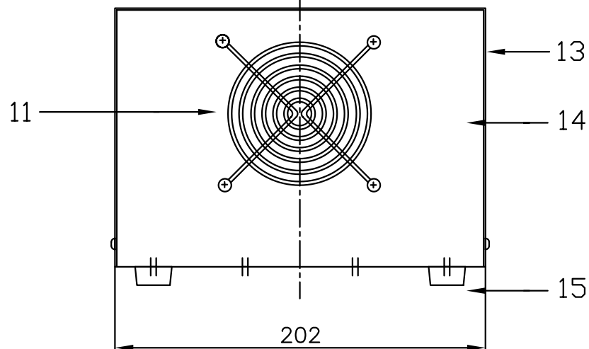
背面図
