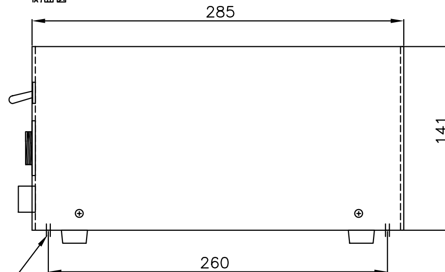
側面図
