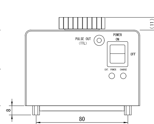
背面 REAR
