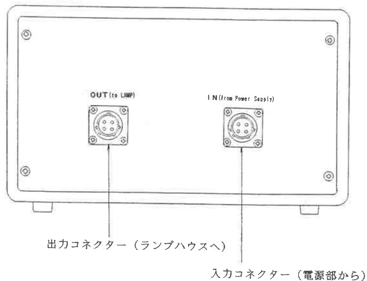
後面図
