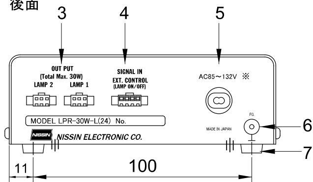
後面
