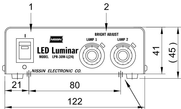
前面
