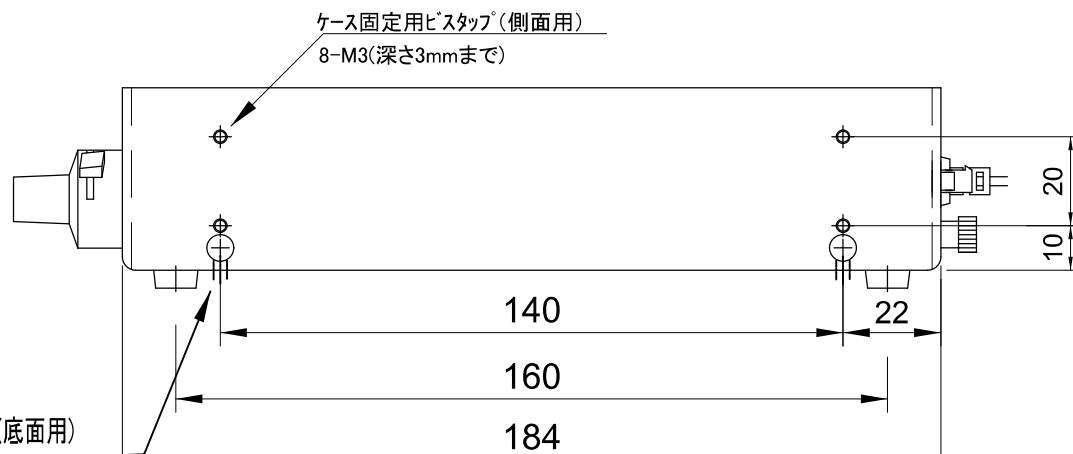
側面
