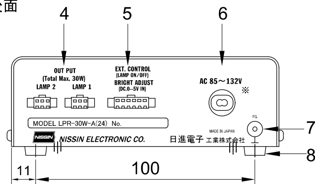
後面
