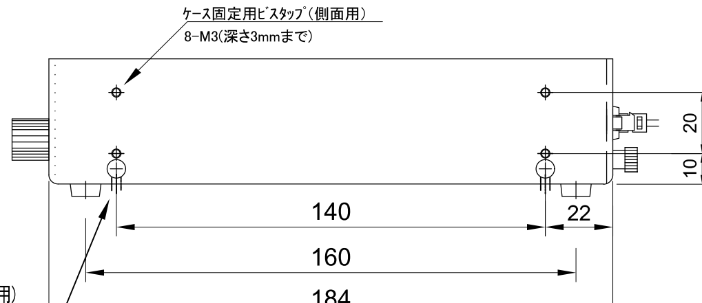
側面
