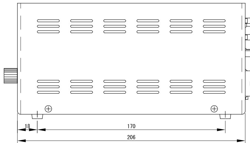
側面
