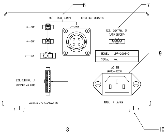
後面
