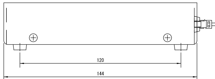
側面
