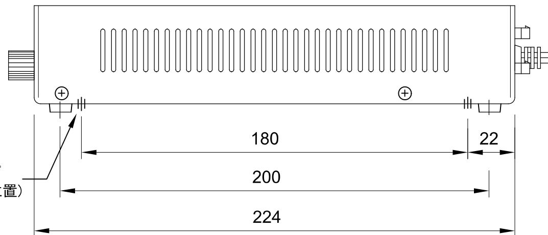
側面
