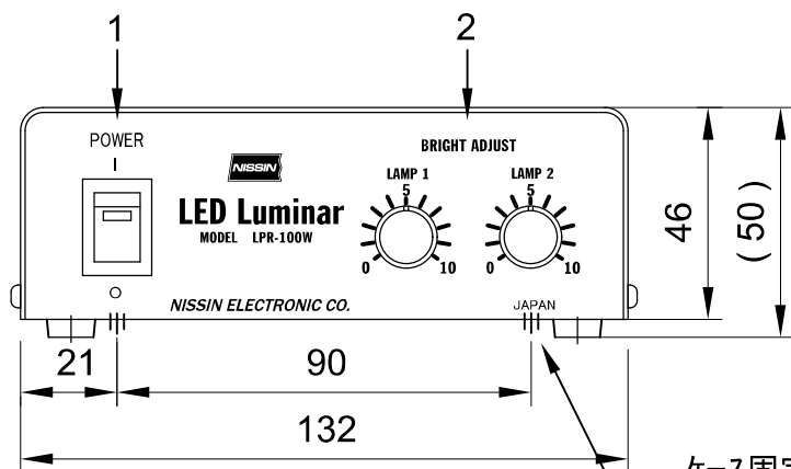
前面
