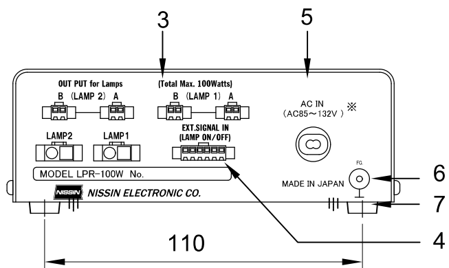
後面
