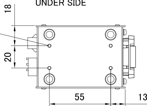
底面 UNDER SIDE
