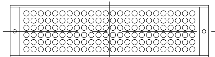
赤,赤外 照明 24個x6列 (素子間P=4mm)
